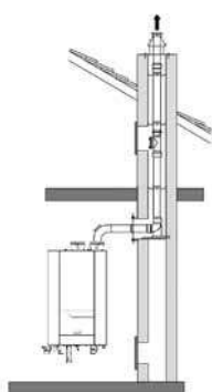
Dimensiones en mm
