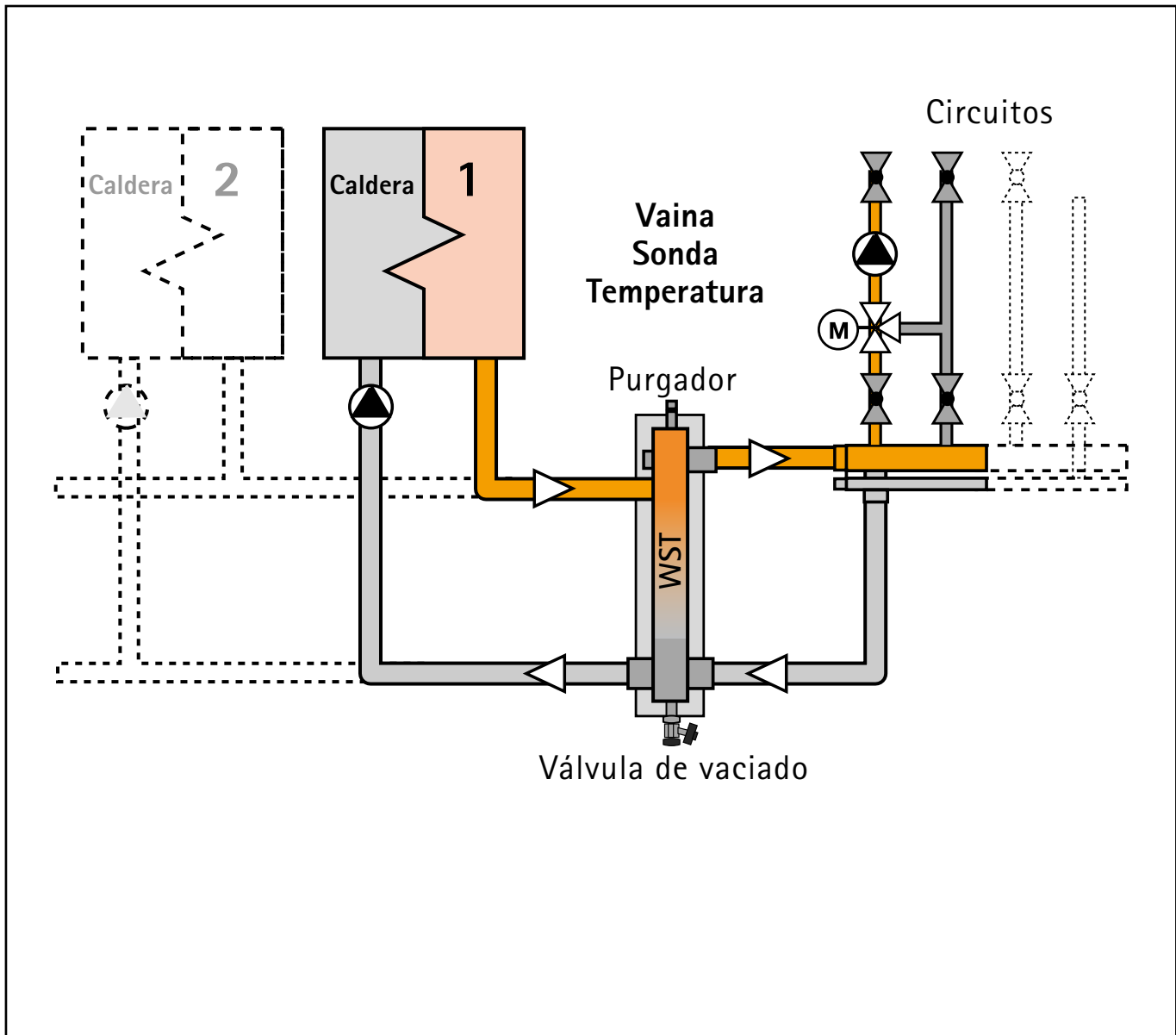
SALTO TÉRMICO EN CIRCUITO SECUNDARIO
