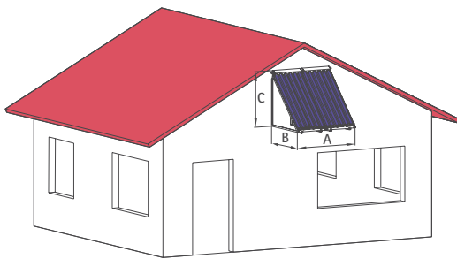
Espacio requerido para un campo de colectores de 1 fila
