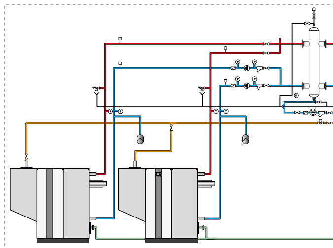
Esquema hidráulico tipo
