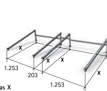
Soporte captador a 15°
