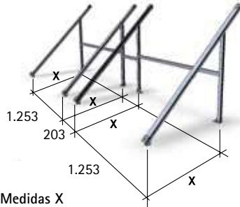
Soporte captador a 30°, 45° y 50°
