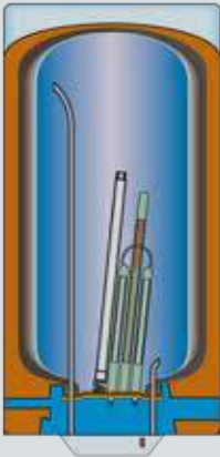
Instalación vertical.
