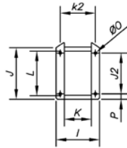
Boca impulsión
