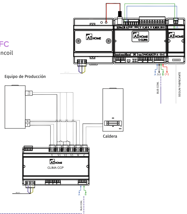
CONEXIÓN CLIMAIAZ Control de climatización (Expansión directa)
