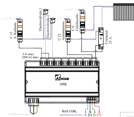
CONEXIÓN OR8 Control de climatización (Radiación hidráulica-eléctrica)
