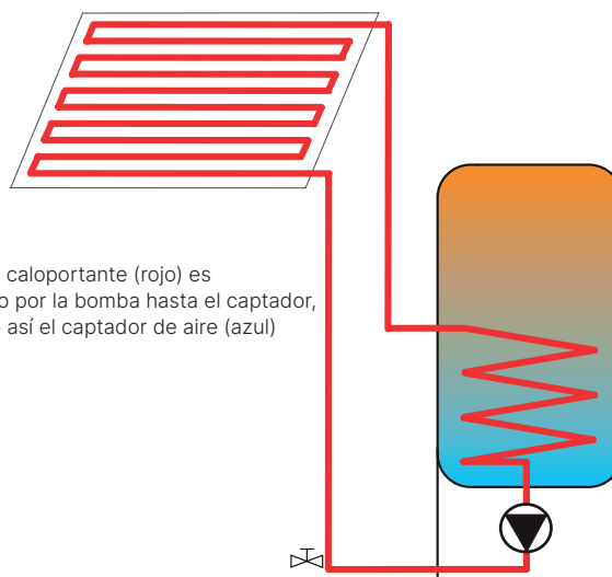
Instalación en funcionamiento / Bomba ON
