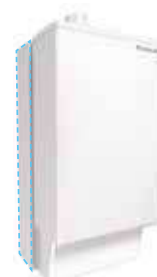
Unidad interior R-32: ACS y suelo radiante
